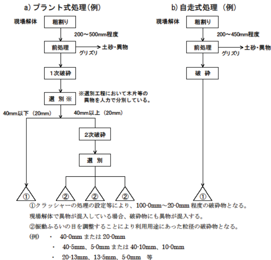
コンクリートがらの破碎処理の例
