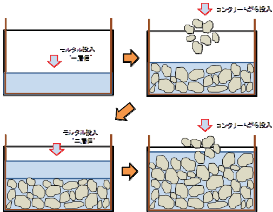
図 4.6 ポストパックドコンクリート方式による2層打設のイメージ図
