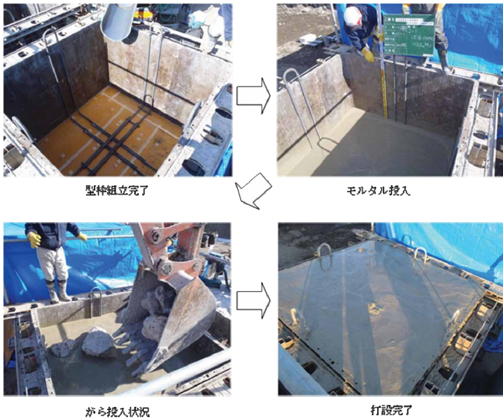
図 4.5 ポストパッドコンクリート方式の打設手順
