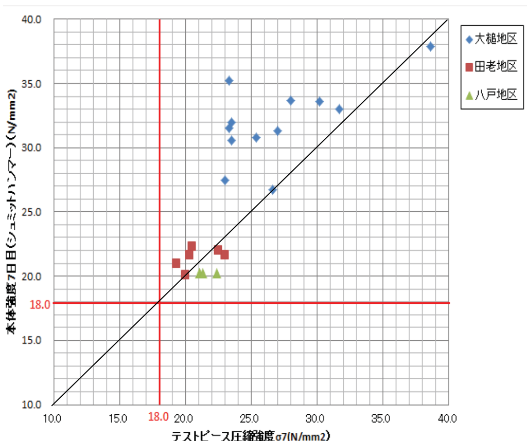
図 6.4 各地区の強度試験結果
